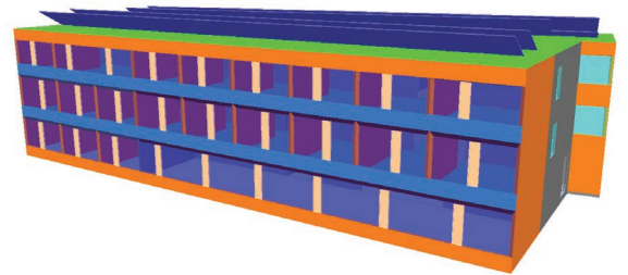
_3D – Simulationsmodell
