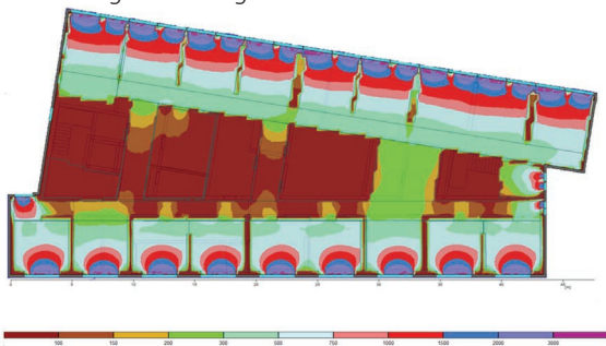
Verteilung der Beleuchtungsstärke im Erdgeschoss
