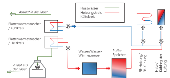
_Prinzipschema der Wärmepumpenanlage
