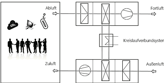
_Prinzip der Lüftungsanlage
